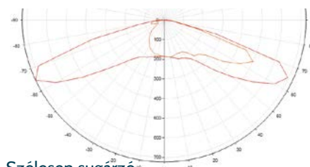
Szélesen sugárzó
