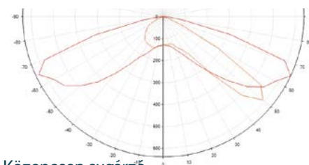
Közepesen sugárzó
